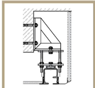
Voorbeeld staalophanging
