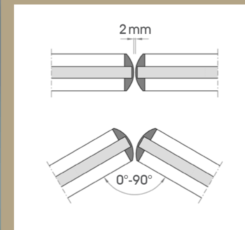
Halfronde spuitgegoten eindkappen zijn bij uitstek geschikt voor veelhoekige scheidingswandconstructies.
