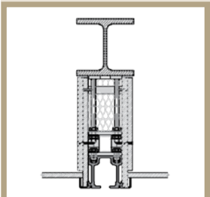
Ophanging aan staal gelast
