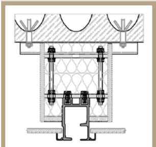
Ophanging aan kanaalplaatvloer
