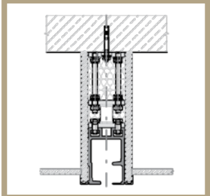
Ophanging aan beton
