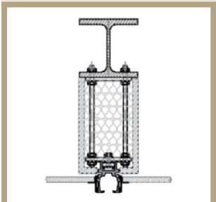
Ophanging aan staalbalk
