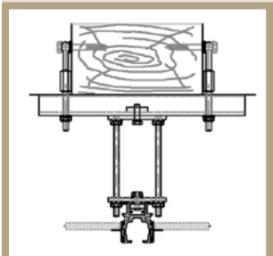
Aan de zijkant van houten balk met montagerails
