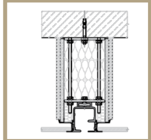
C-profiel, dubbele afscheiding, montage onder betonlatei
