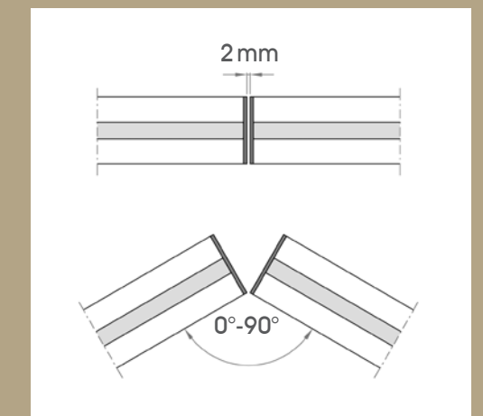
Platte rvs-eindkappen voor een vormvaste overgang van de aluminiumprofielen
