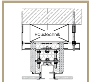
Voorbeeld kokerprofiel
