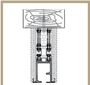
Ophanging aan houten balk
